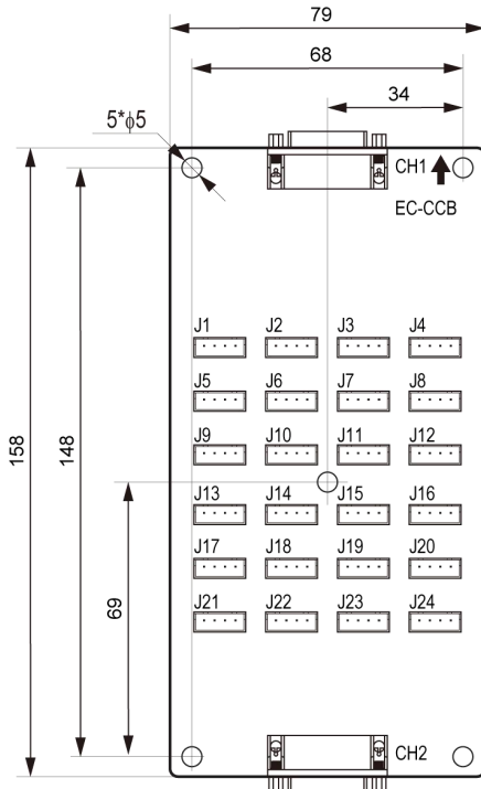
图 9-2 指令板安装尺寸
