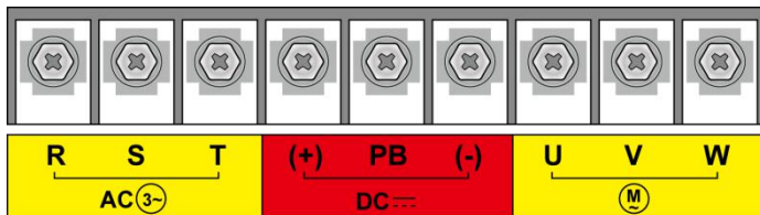
图 4-4 EC160A 电梯智能整体机主回路端子排的布局(18.5kW~30kW)
