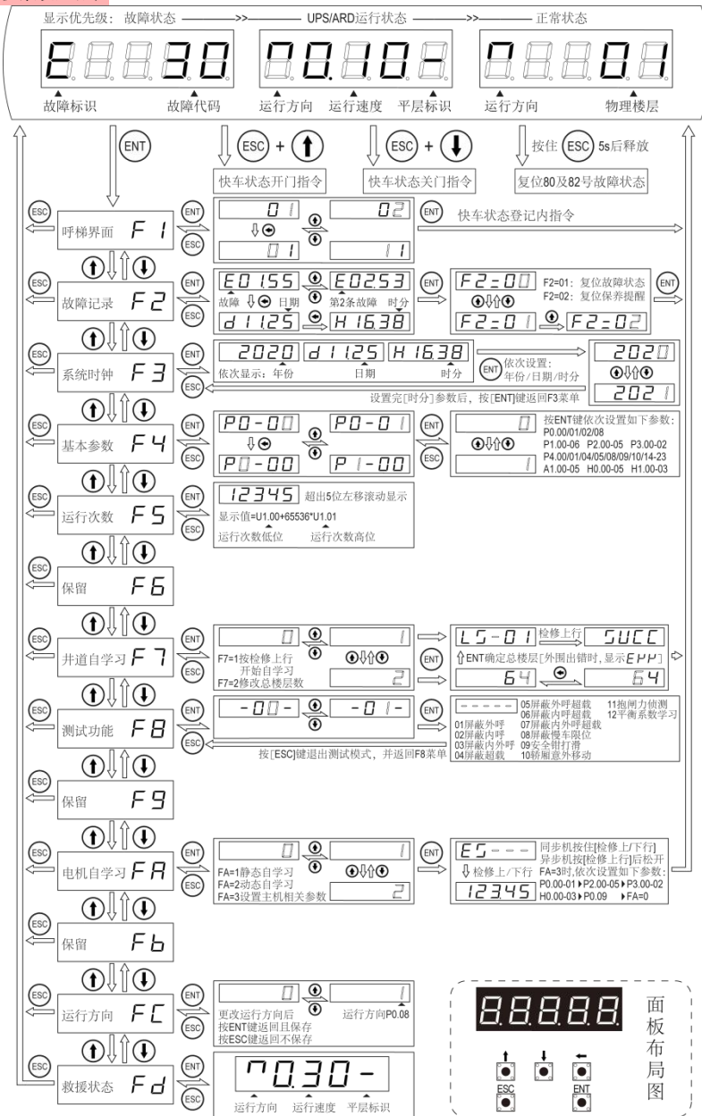
图 8-2 操作流程图
