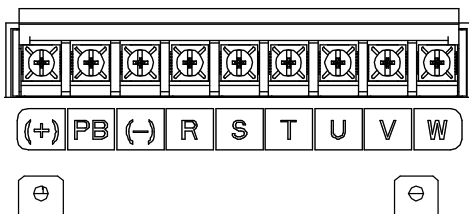
图 4-4 380V 7.5~18kW 主回路端子示意图
