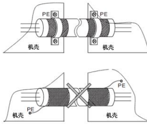
图 4-8 360 度环接示意图
