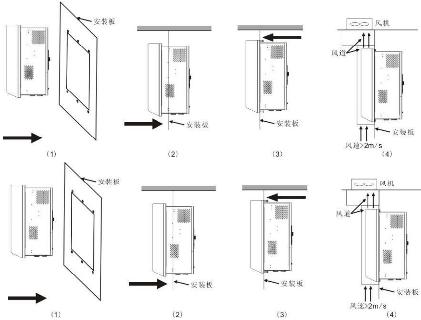
图 4-2 安装示意图
