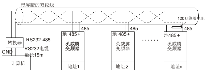
图 11-4 菊花接法运用图
