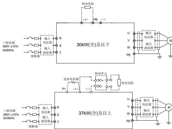
图 4-3 380V 主回路接线图
