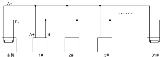
图 11-3 菊花简化接线图
