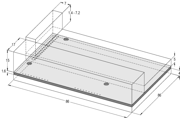
图 A-2 EC-TX-103 通讯卡外形尺寸图（单位：mm）
