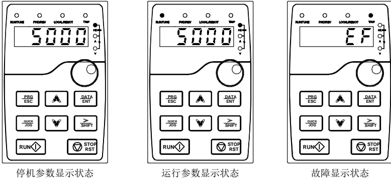
图 5-2 状态显示示意图
