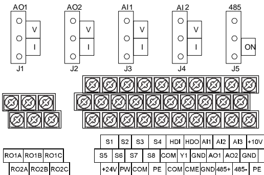
图 4-10 控制端子示意图
