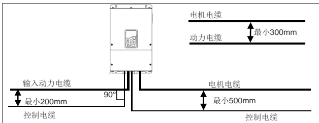
图 D-3 布线距离
