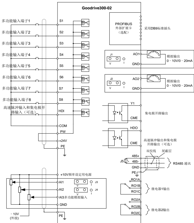
图 4-9 控制回路接线图
