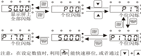
图 5-5 查看参数示意图
