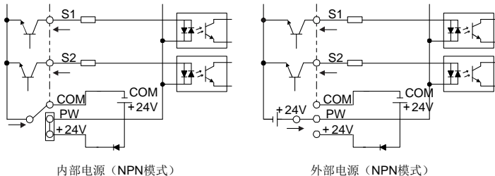
图 4-12 NPN 模式示意图
