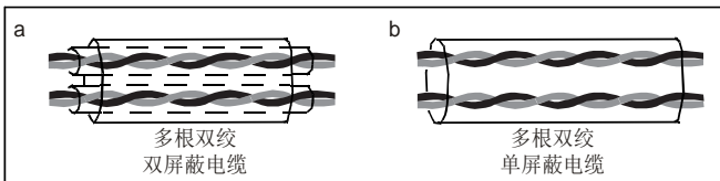
图 D-2 动力电缆布线
