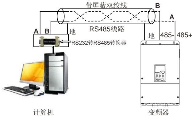
图 11-1 RS485 单机应用时的物理接线图
