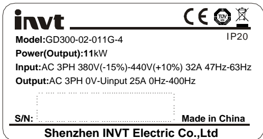
图 3-3 产品铭牌
