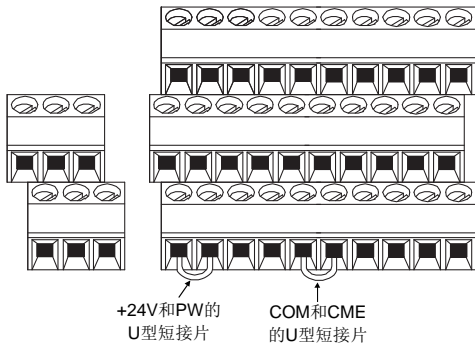
图 4-11 U 型短接位置示意图
