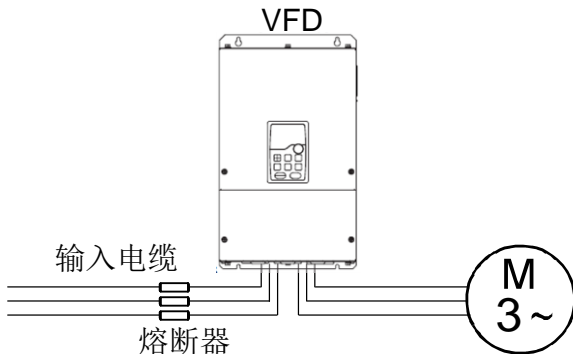
图 4-14 熔断器配置图
