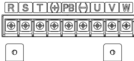
图 4-5 380V 22~30kW 主回路端子示意图
