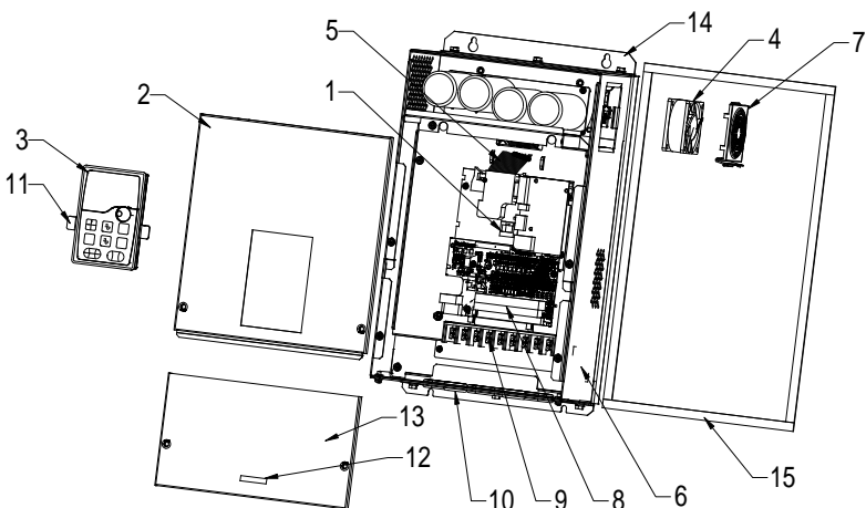
图 3-5 产品结构示意图
