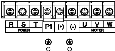
图 4-6 380V 37~55kW 主回路端子示意图
