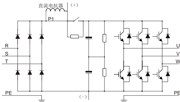
图 3-2 380V（大于 37kW（含））主回路简图
