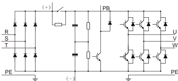
图 3-1 380V（小于 30kW（含））主回路简图
