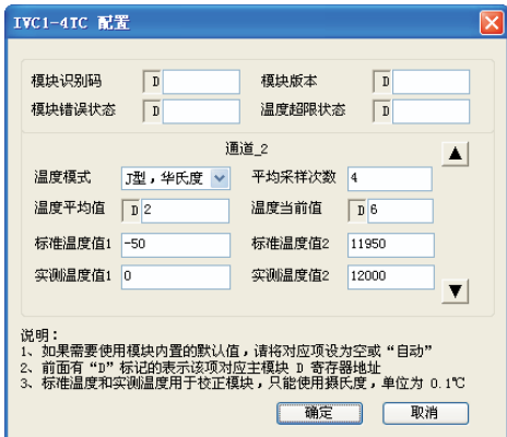
图 4-6 模块第 2 通道设置更改界面
