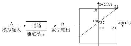
图 3-1 IVC1-4TC 的通道特性示意图
