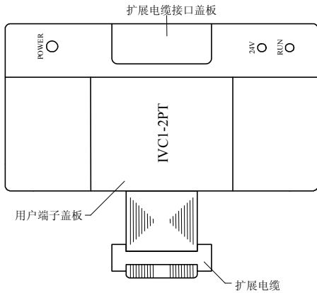
图 1-1 模块接口外观图
