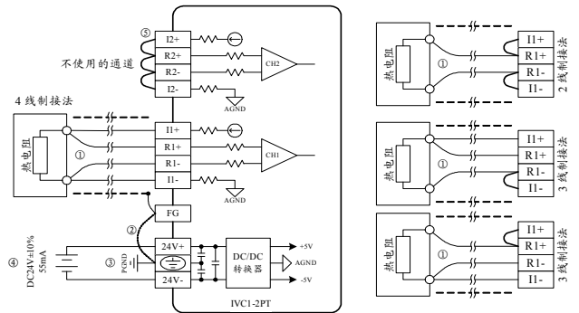
图 1-4 用户端子布线示意图
