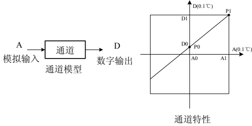
图 3-1 IVC1-2PT 通道特性示意图
