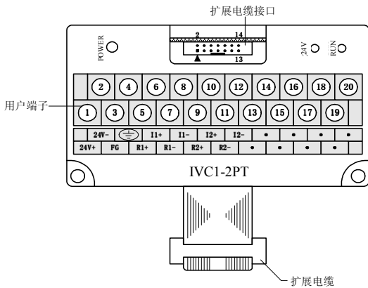
图 1-2 接模块接口端子图
