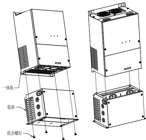
图 B-7 底座安装示意图
