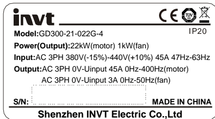
图 1-1 产品铭牌
