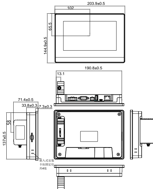
图 B-15 触摸屏安装尺寸（单位：mm）
