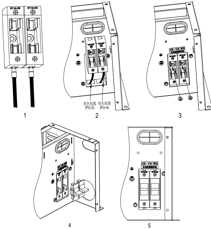
图 B-2 熔断器底座安装示意图
