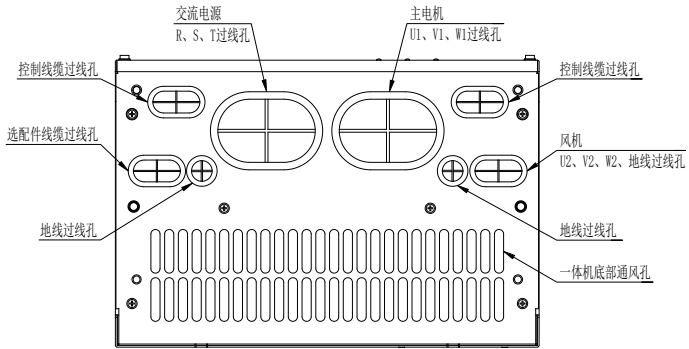
图 4-6 AC380V 45~ 90kW 仰视
