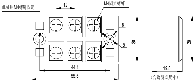
图 B-4 转接端子尺寸 (单位 mm)
