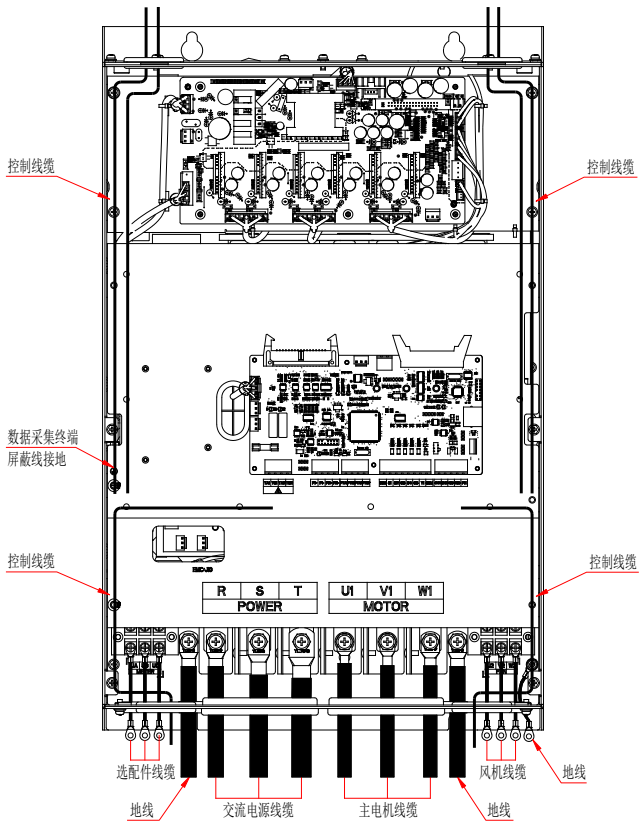
图 4-7 AC380V 45~ 90kW 正面接线示意图
