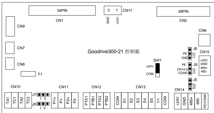
图 2-4 控制回路布局示意图
