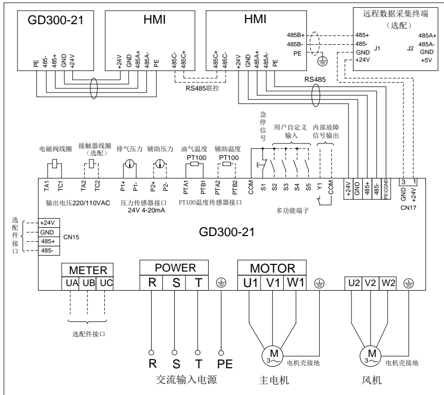
图 4-1 空压机一体机系统接线
