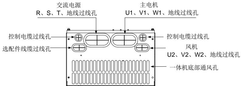
图 4-4 AC380V 30~37kW 仰视
