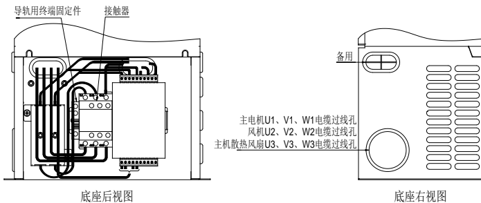
图 B-8 底座选配件背面接线示意图
