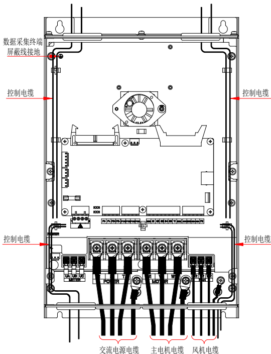
图 4-3 AC380V 15~22kW 正面接线示意图
