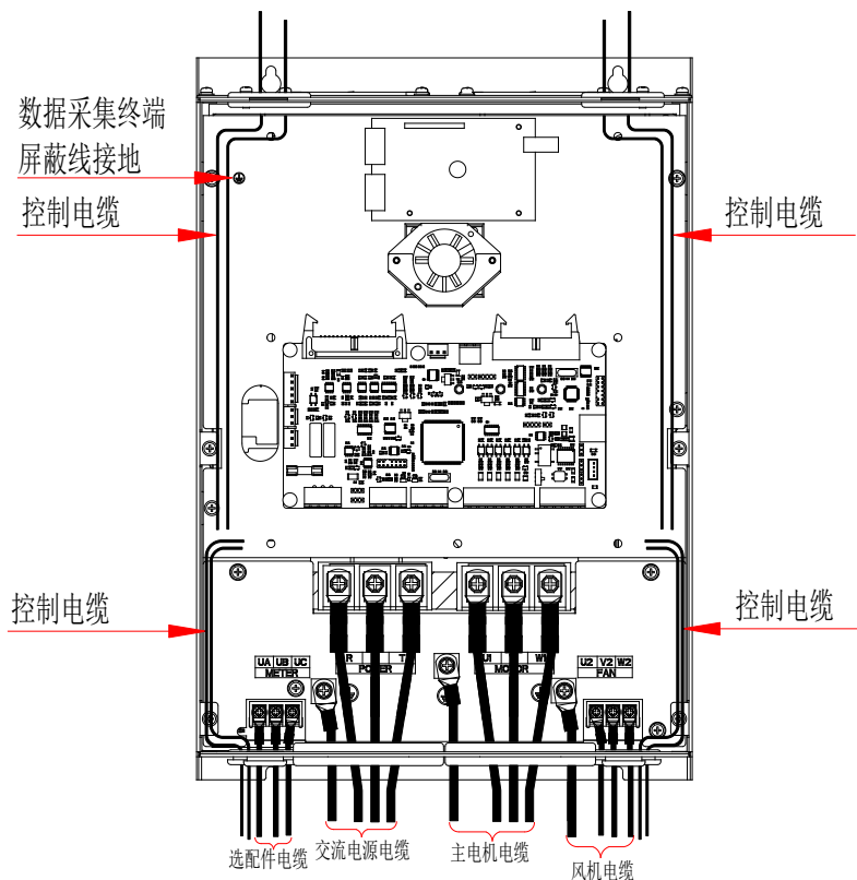
图 4-5 AC380V 30~37kW 正面接线示意图
