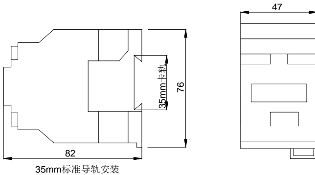
图 B-3 接触器尺寸 (单位 mm)
