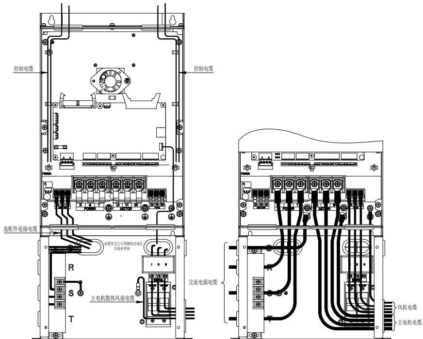
图 B-10 控制回路和主回路接线示意图
