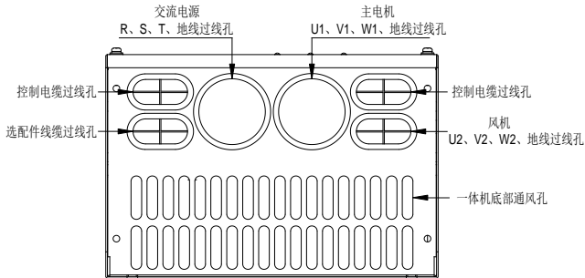
图 4-2 AC380V 15~22kW 仰视
