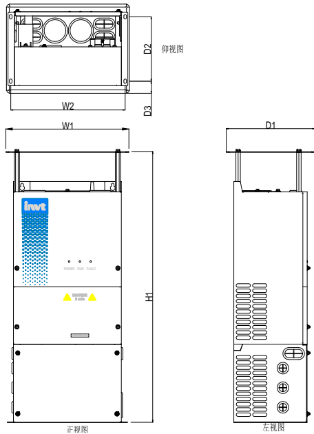
图 A-3 AC220V 7.5~45kW/AC380V 15~90kW 落地安装 (带顶盖) 示意图
