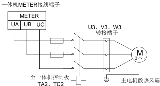
图 B-1 接触器组件电气接线
