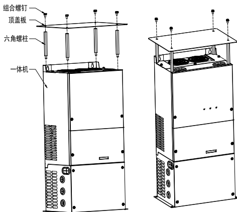
图 B-6 防滴水顶盖安装示意图
