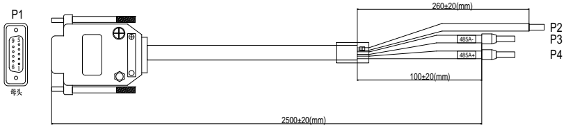
图 B-14 触摸屏通讯线示意图
