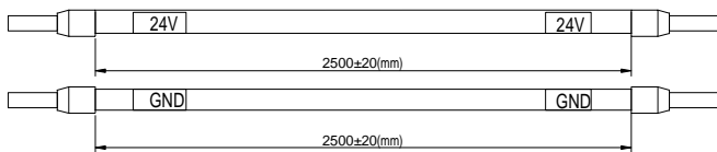
图 B-13 触摸屏电源线示意图
