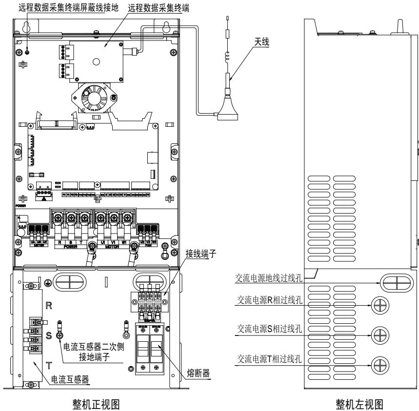
图 B-9 底座选配件安装示意图
