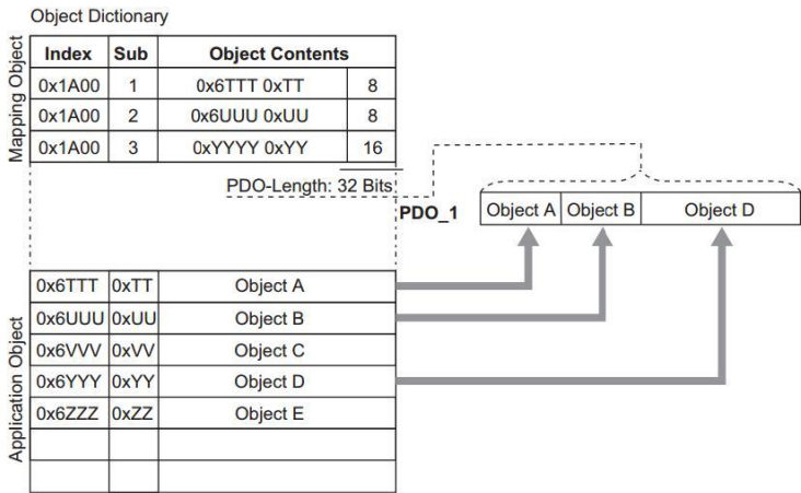
图 9-3 PDO 映射示例
