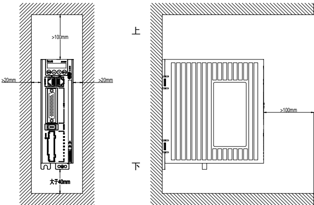
图 3-1 单台安装
