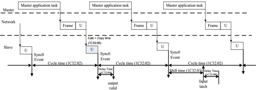
图 9-5 DC 模式时序图
