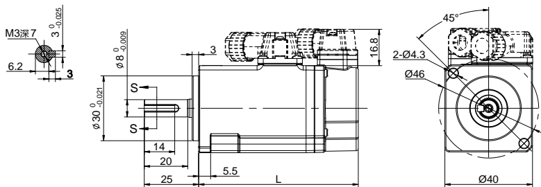
图 3-3 40 机座外形及安装尺寸 (单位: mm)
