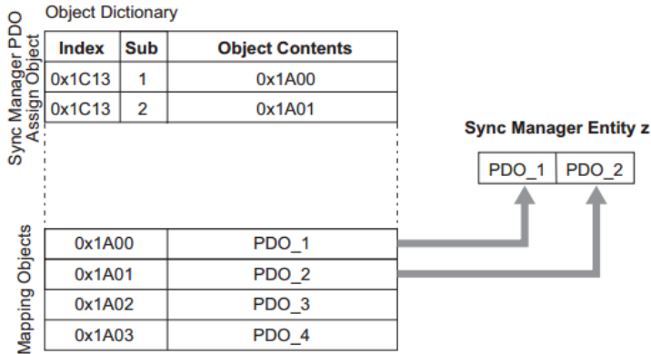
图 9-4 PDO 分配示例
