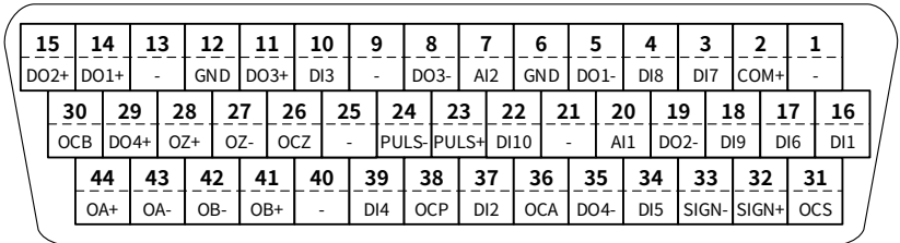
CN1 插头引脚号及信号代码
