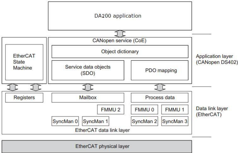
图 9-1 CoE 参考模型
