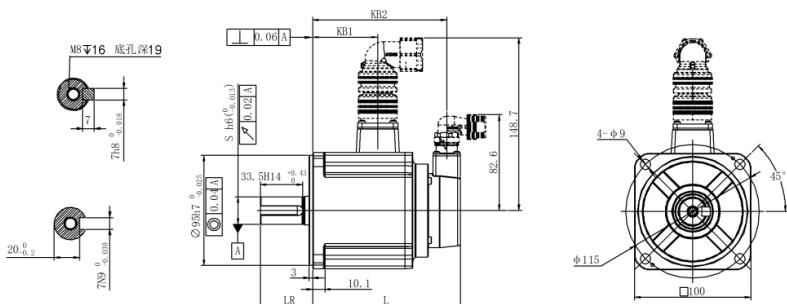
图 3-6 100 机座外形及安装尺寸 (单位: mm)
