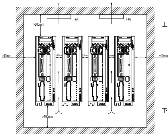
图 3-2 多台安装
