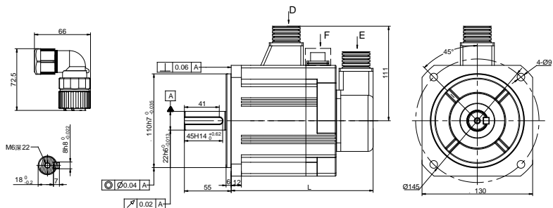
图 3-7 130 机座外形及安装尺寸 (单位: mm)
