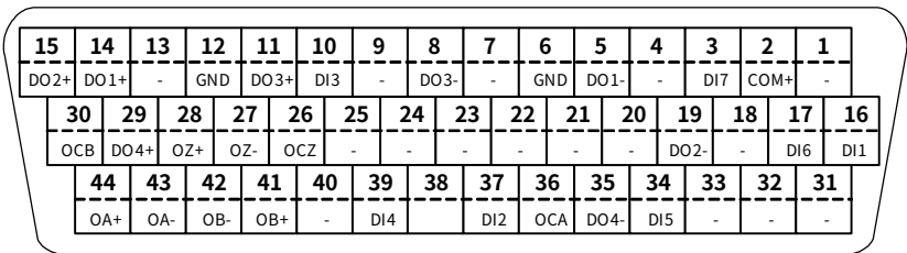
图 5-2 EtherCAT 总线型接口
