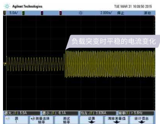
V/F控制模式, 2Hz突加100%负载的电流波形
