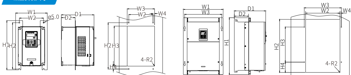
法兰安装尺寸
