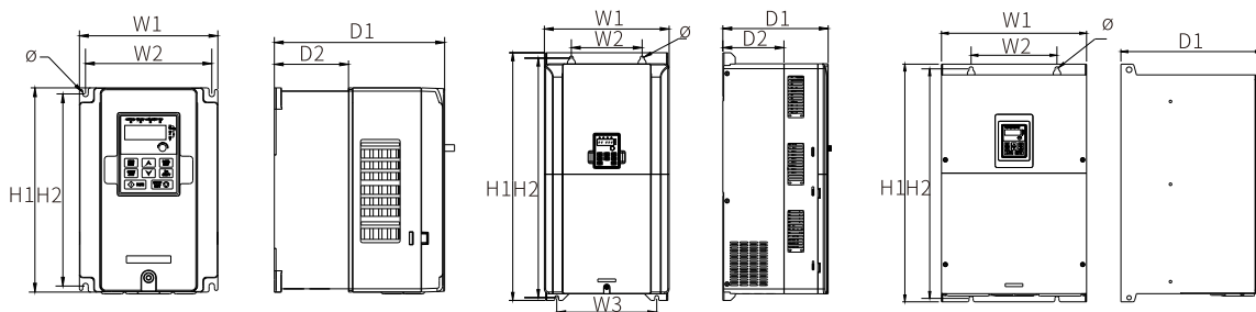
壁挂安装尺寸
