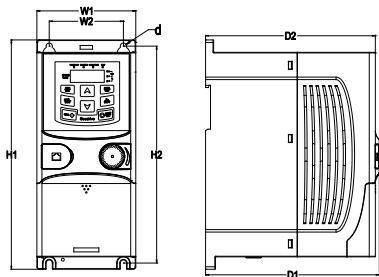
图 B-4 0.75~2.2kW 壁挂安装
