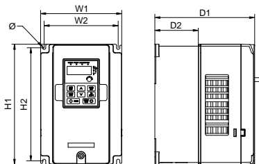
图 B-6 三相 220V 1.5~7.5kW/三相 400V 4~37kW 壁挂安装
