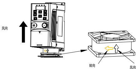
图 6-1 单相 230V 2.2kW（含）以下机器风扇维护
