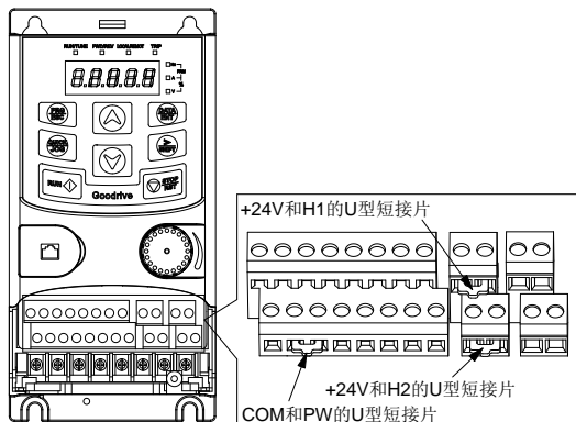
图 3-13 U 型短接位置
