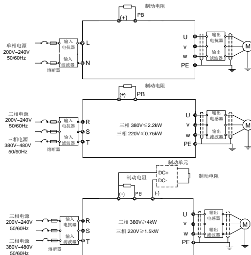
图 3-3 主回路接线
