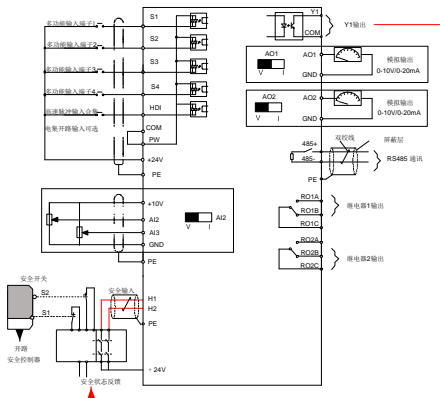
图 3-10 三相 230V 1.5kW (含) / 三相 400V 4kW (含) 以下控制回路接线
