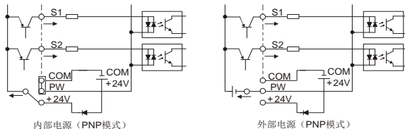
图 3-15 PNP 模式
