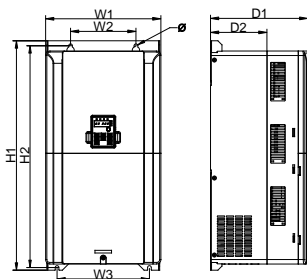
图 B-7 三相 400V 45~75kW 壁挂安装
