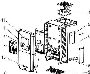
图 2-4 三相 380V 4kW（含）以上产品结构
