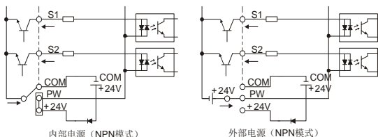
图 3-14 NPN 模式
