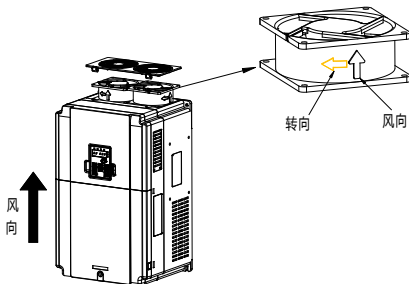
图 6-2 三相 400V 4kW（含）以上机器风扇维护
