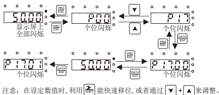
图 4-6 查看参数
