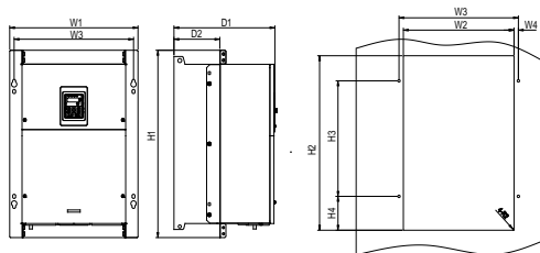
图 B-11 三相 400V 90~110kW 法兰安装
