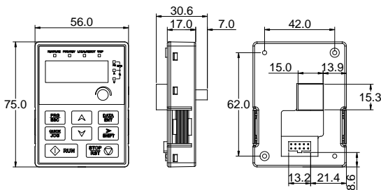
图 B-1 键盘外形 (单位: mm)
