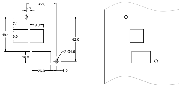
图 B-2 键盘无支架开孔 (单位: mm)
