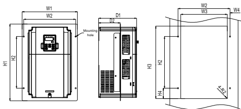
图 B-10 三相 380V 18.5~75kW 法兰安装
