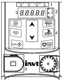
图 4-1 贴膜键盘
