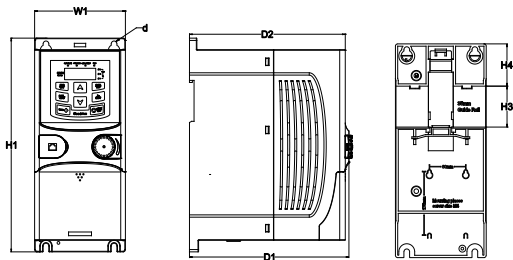
图 B-5 单相 230V 2.2kW(含)/三相 230V 0.75 kW (含)/三相 400V 2.2kW(含)以下导轨安装
