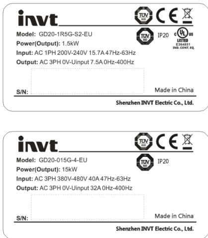
图 2-1 产品铭牌
