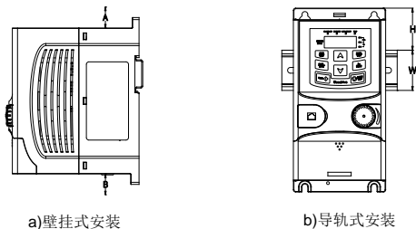
图 3-1 安装方式
