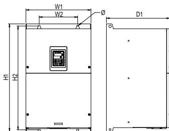
图 B-8 三相 400V 90~110kW 壁挂安装
