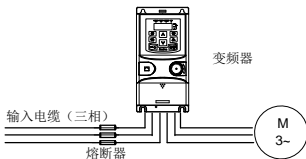
图 3-17 熔断器配置
