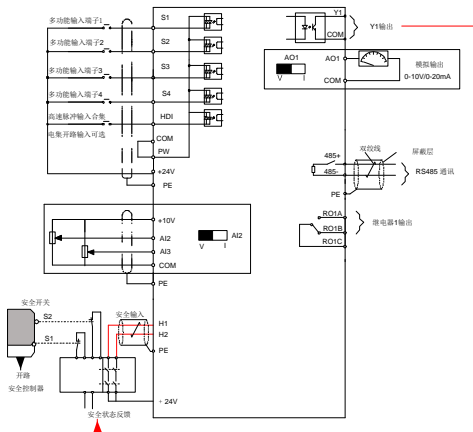
图 3-9 单相 230V 2.2kW（含）/三相 230V 0.75kW（含）/三相 400V 2.2kW（含）以下控制回路接线
