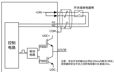
图 3-16 STO 功能电路
