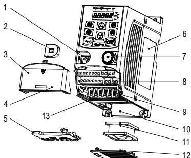
图 2-3 三相 400V 2.2kW（含）以下产品结构
