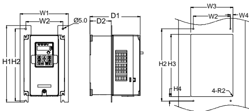
图 B-9 三相 400V 4~75kW/三相 230V 1.5~7.5kW 法兰安装
